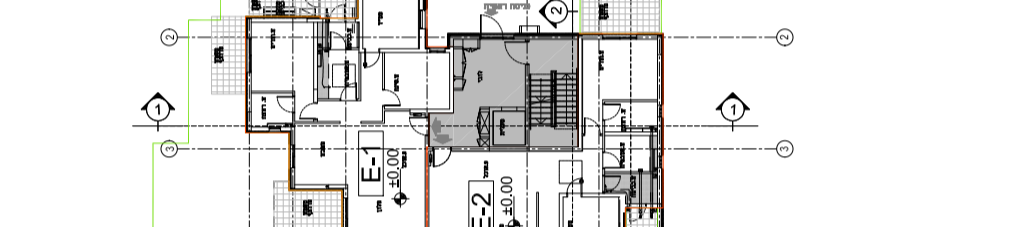
תכנית דירת ג' סופוס E.F. תכנית קומת קרקע
